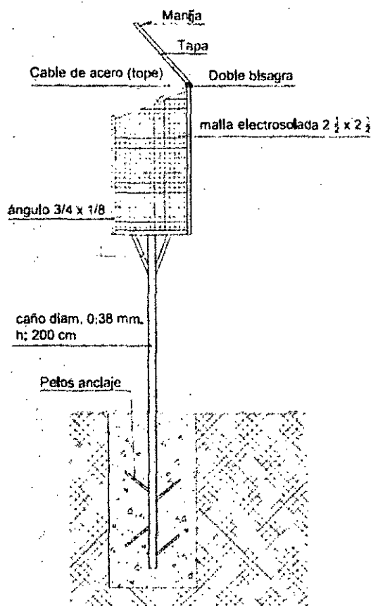
CORTE TRANSVERSAL
