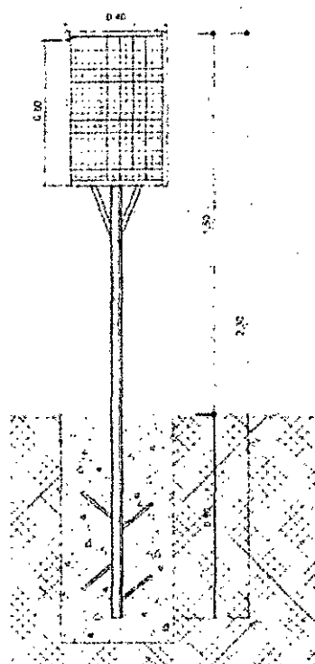
VISTA B
