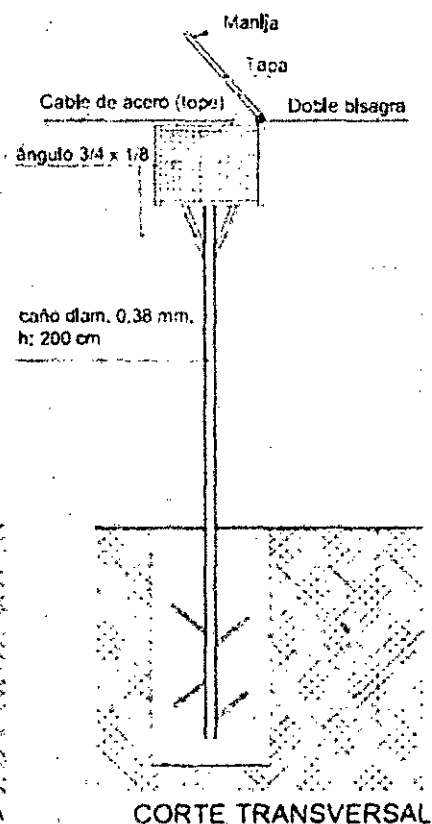
CORTE TRANSVERSAL
