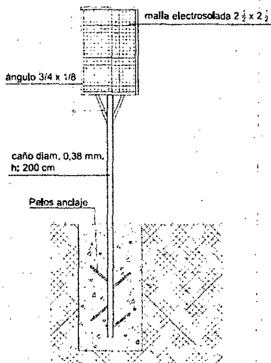
CORTE TRANSVERSAL
