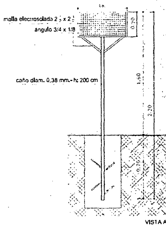
VISTA A
